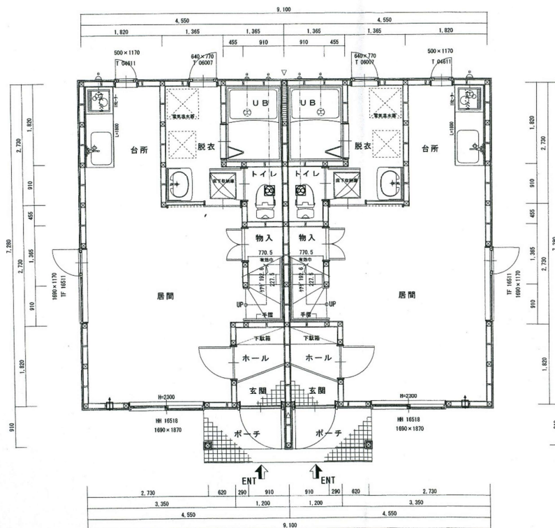
1 階平面図 1/50
