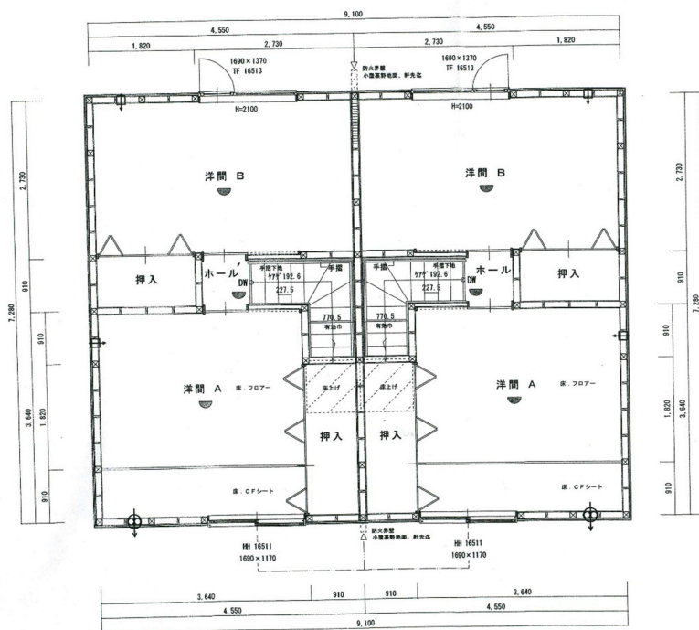
2 階平面図 1/50
