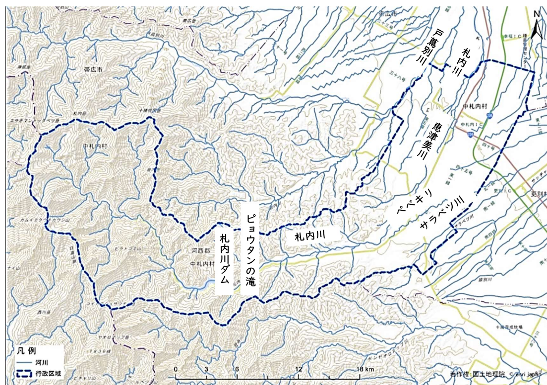
図 2-4 水系図
