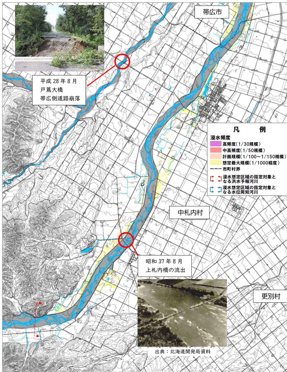
図 2-17 浸水深 50 センチメートル以上の頻度マップ（床上浸水が発生するおそれのある頻度）
