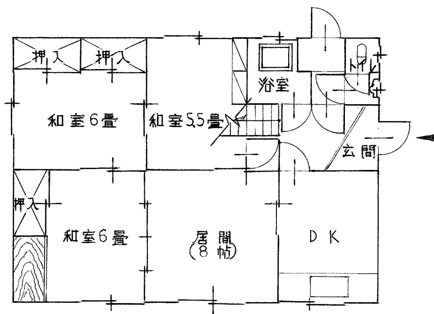
1 階間取り図
