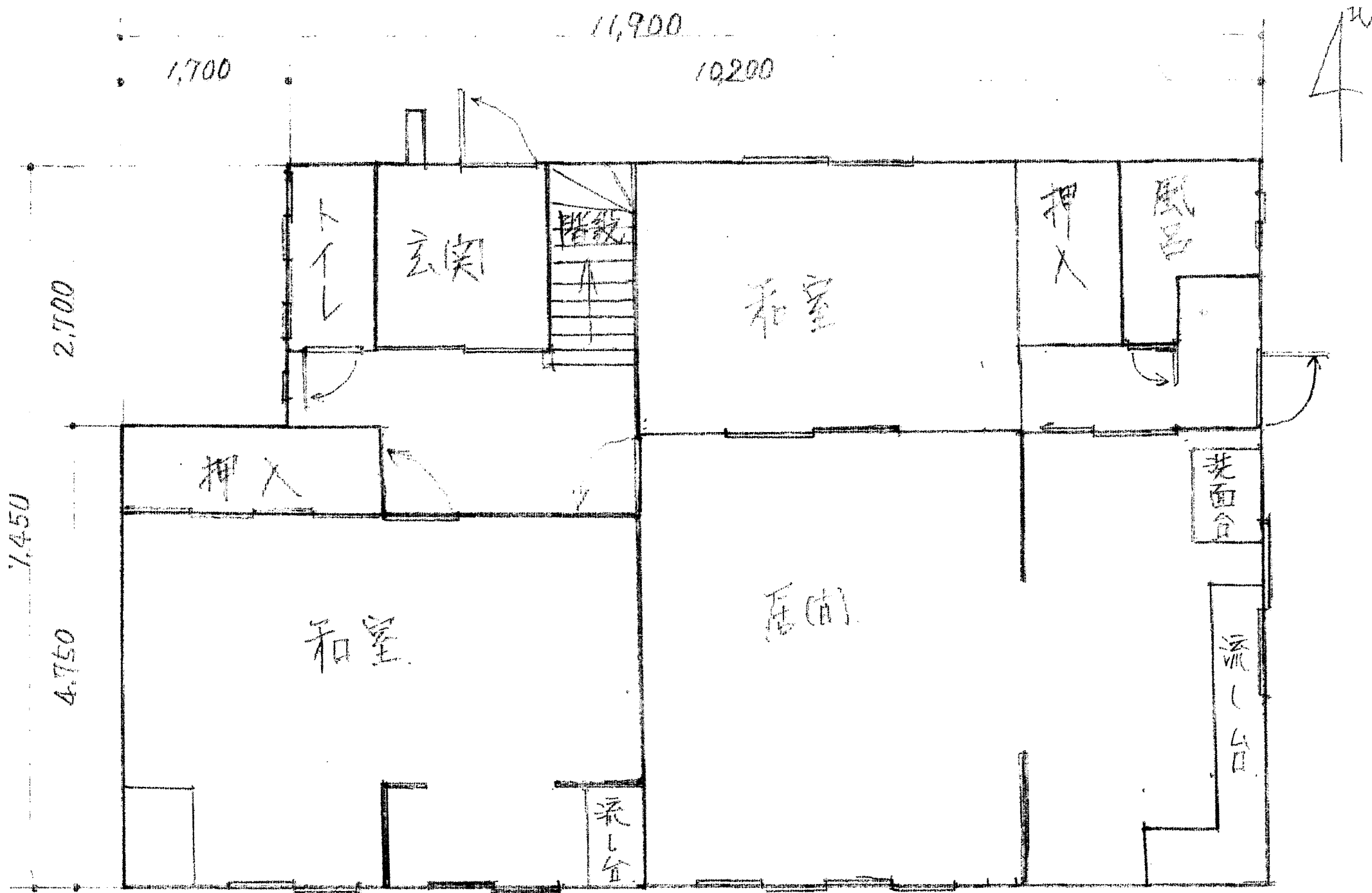
1 階 平面図
