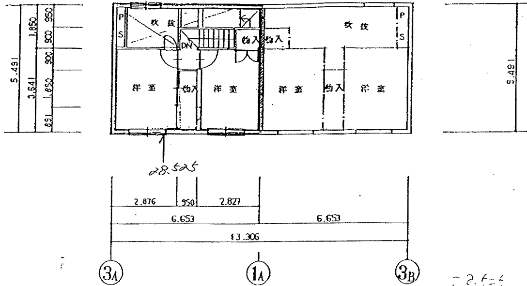
2 階平面図
