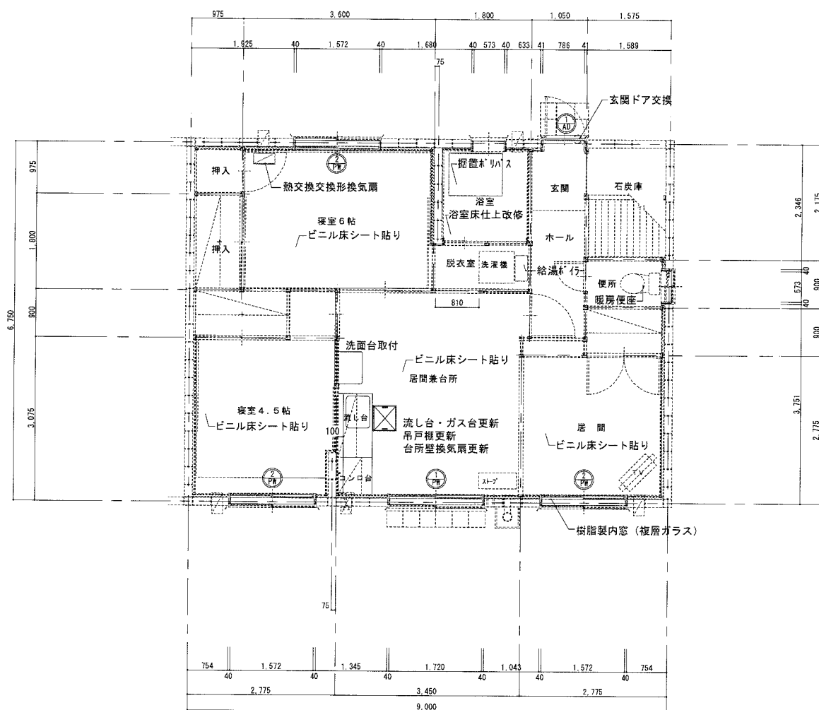
H30年度改修 元札内団地1, 2棟 改修後2LDK平面詳細図 (60.75m 2 )
