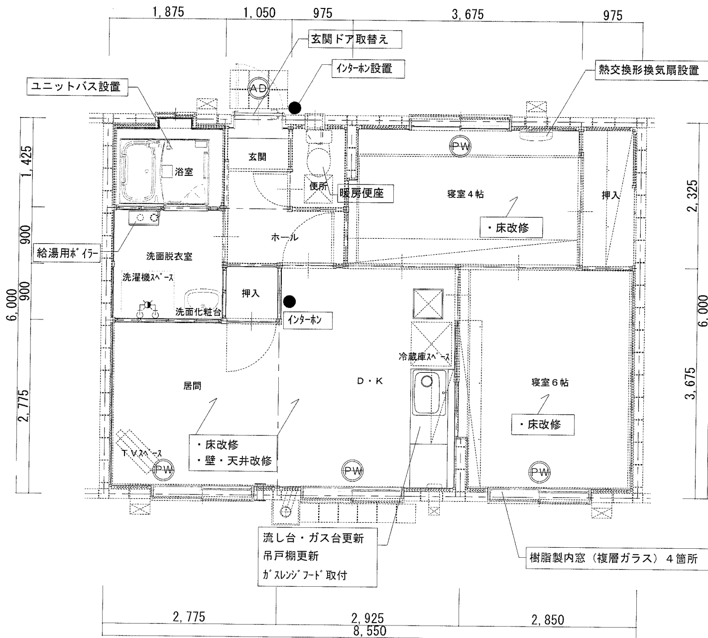
改修後 2LDK 平面詳細図 (51.3㎡)
