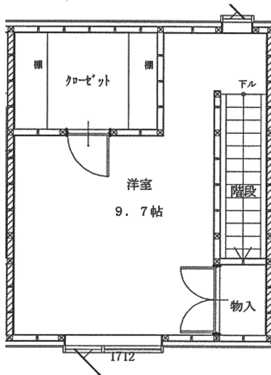
2階平面図
