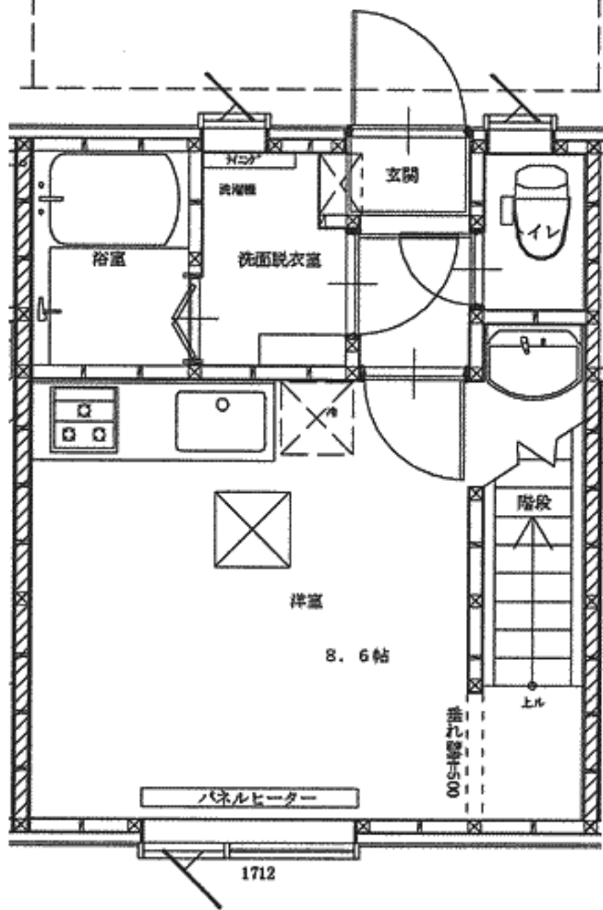
1階平面図
