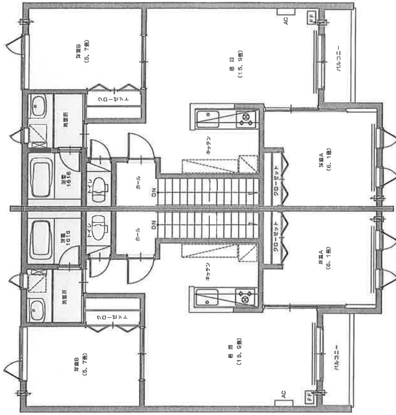
B 棟 2 階 平面図
