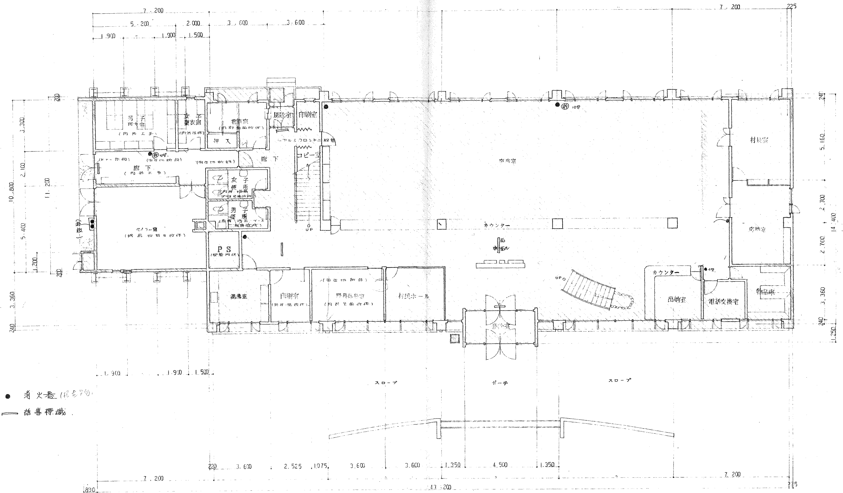
1 階 平面図
