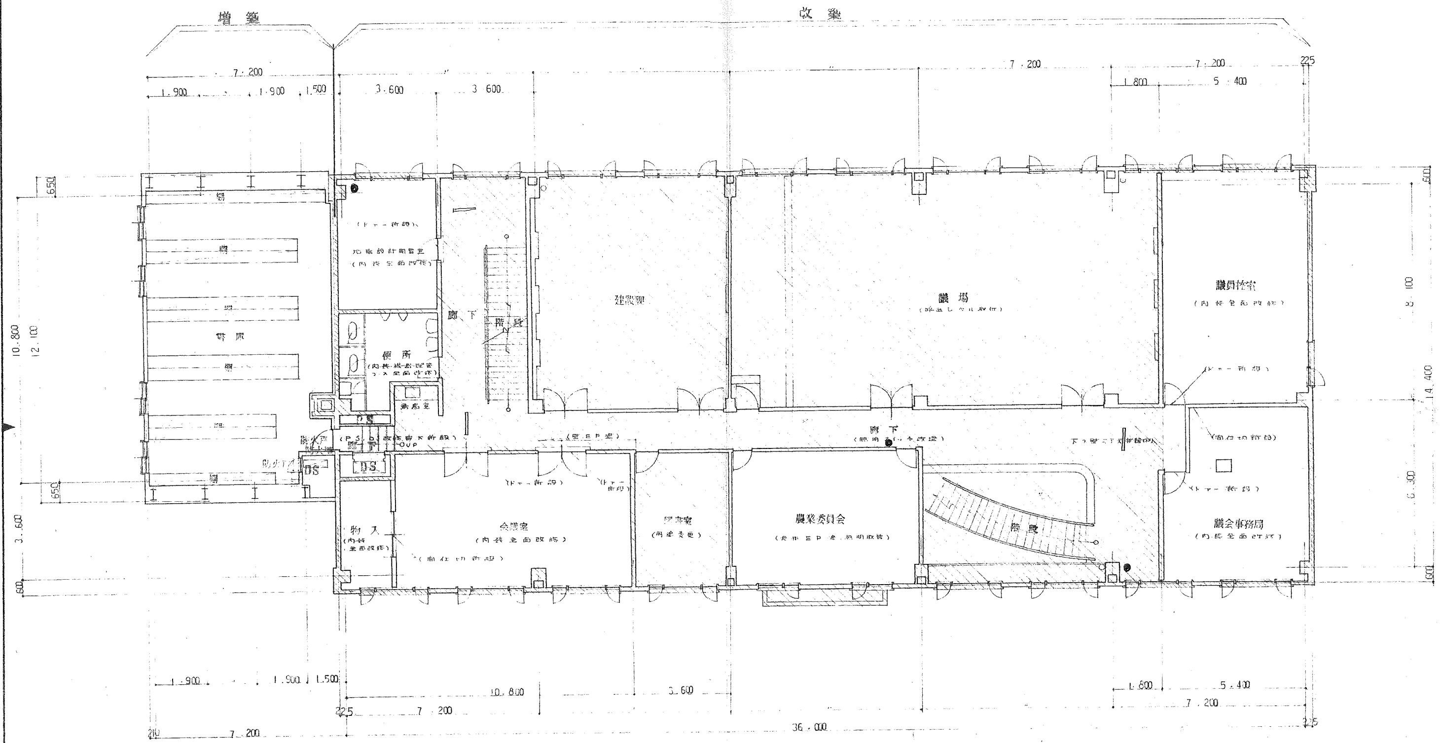
2 階 平 面 図
