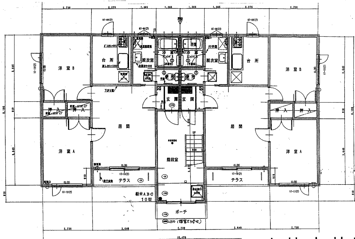
1階 平面図
